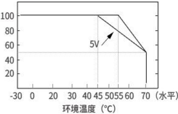
温度降额曲线
